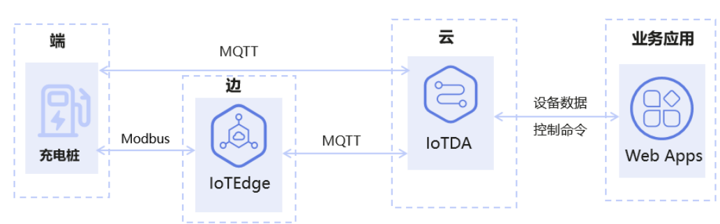
图 3-9 智慧充电桩场景参考架构图
