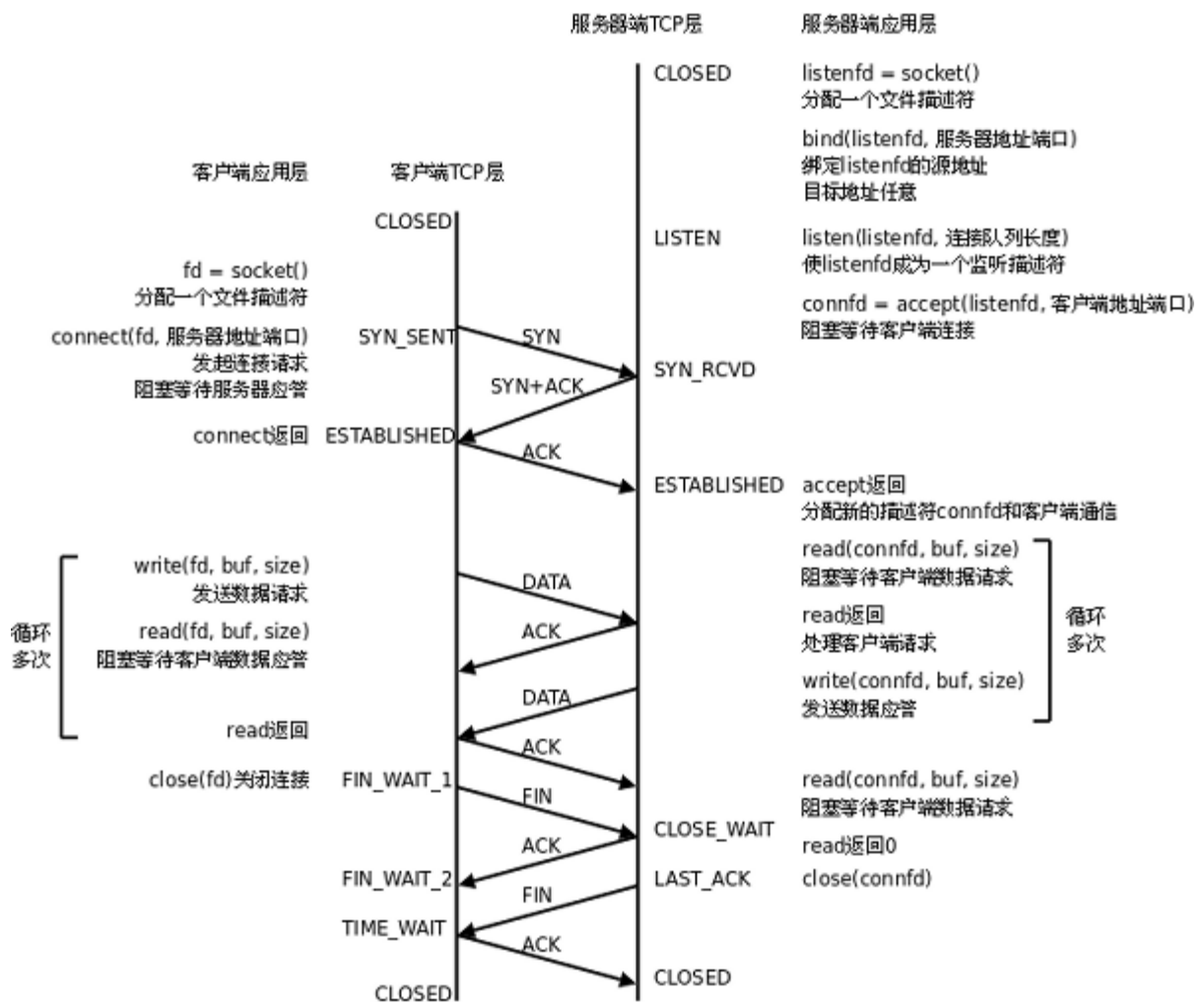
图 37.2. TCP协议通讯流程
