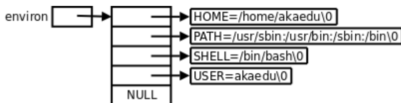
图 30.3. 环境变量
