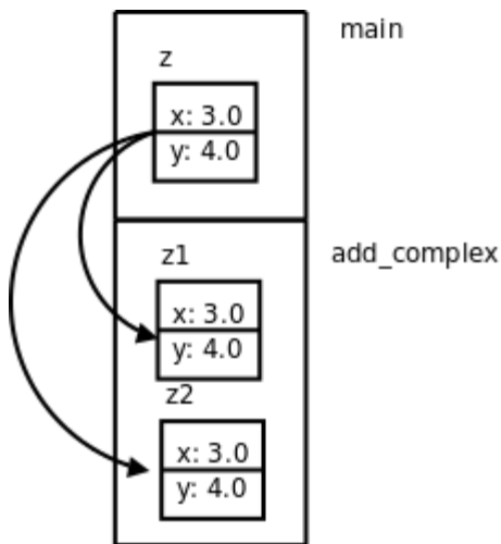
图 7.2. 结构体传参
