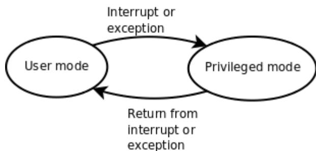
图 17.7. 处理器模式
