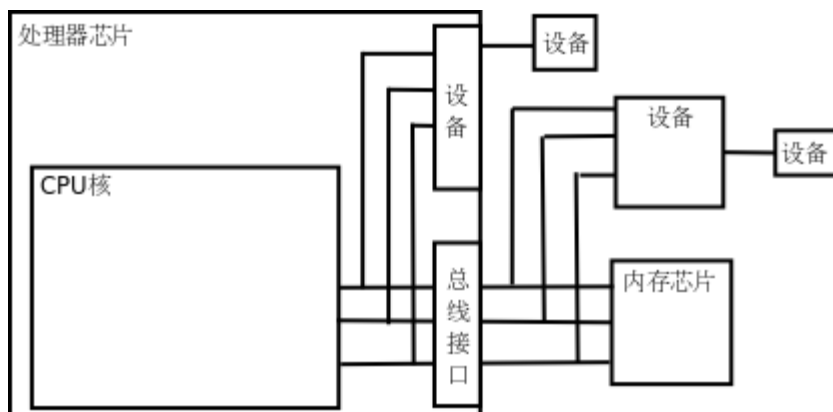
图 17.4. 设备
