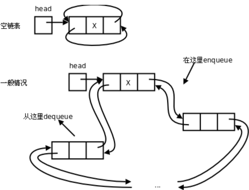
图 26.7. 环形链表
