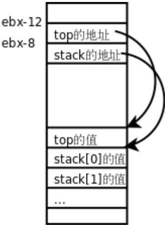
图 20.3. 间接寻址
