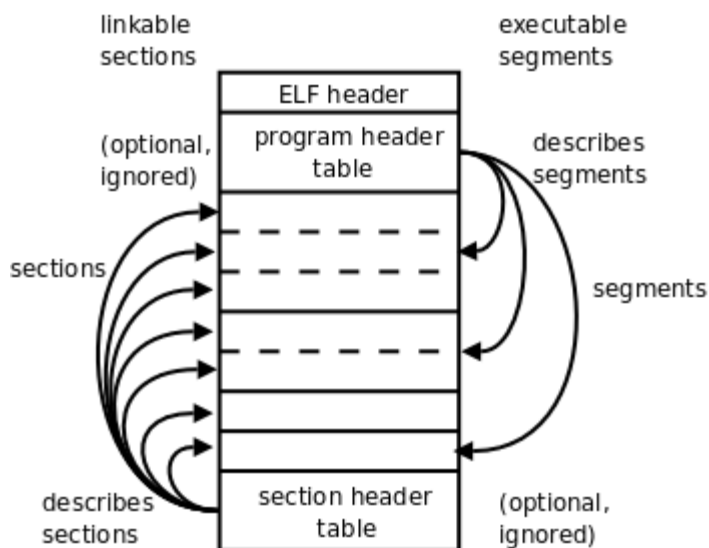
图 18.1. ELF文件
