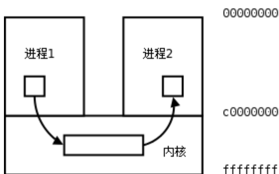
图 30.6. 进程间通信
