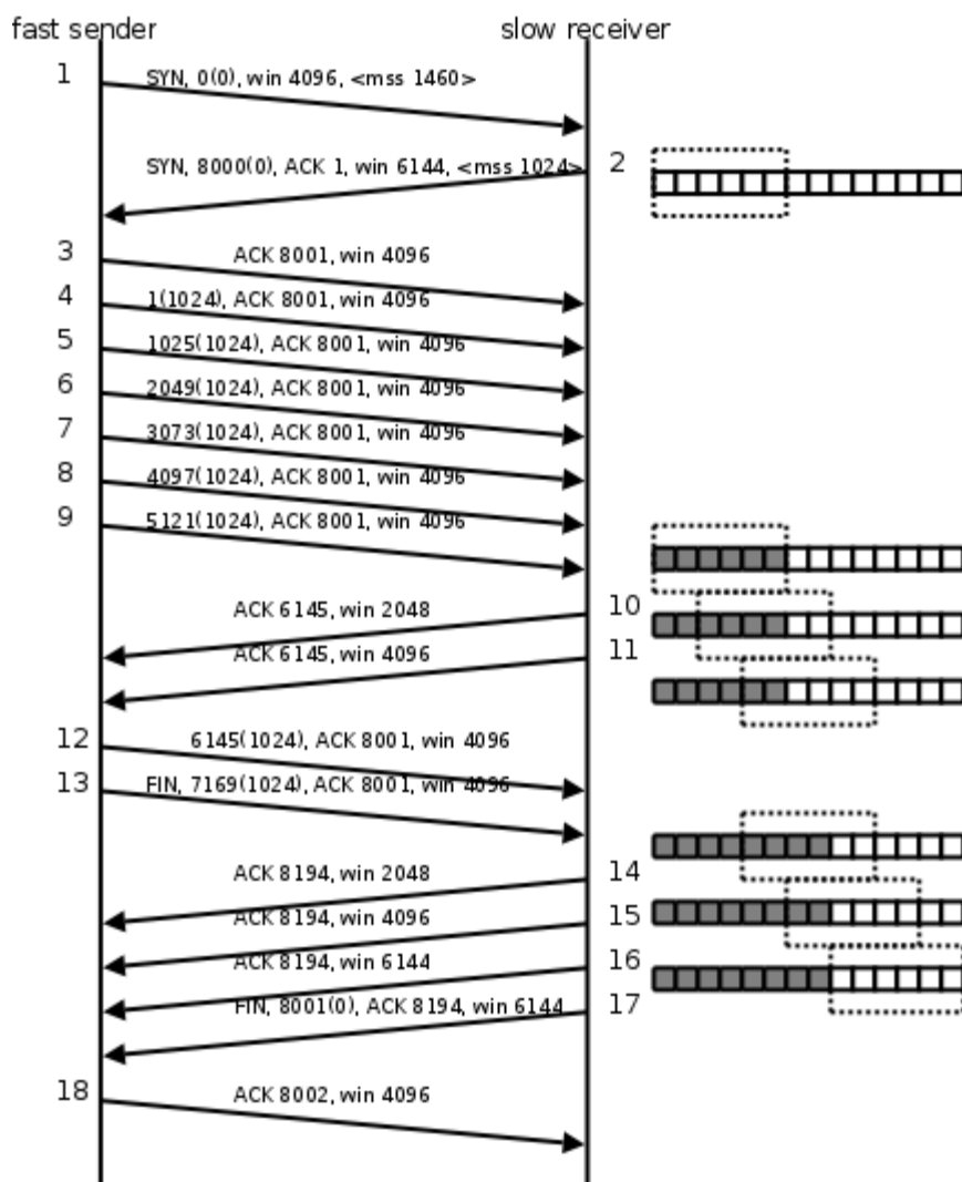
图 36.14. 滑动窗口
