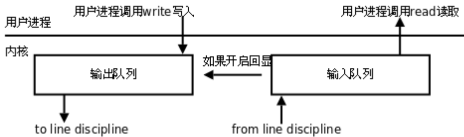
图 34.2. 终端缓冲
