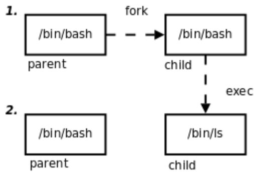
图 30.1. fork/exec
