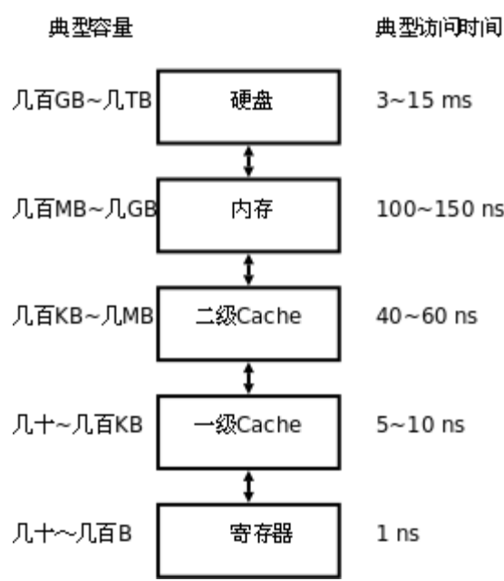
图 17.8. Memory Hierarchy
