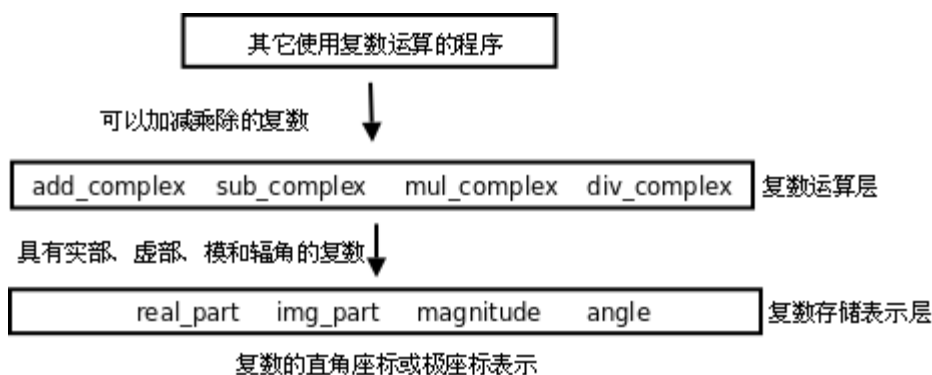
图 7.3. 数据抽象
