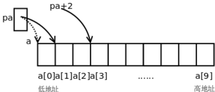
图 23.3. 指针与数组
