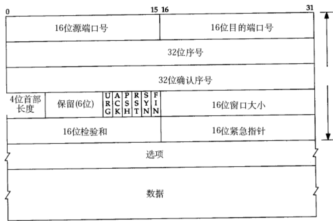
图 36.12. TCP段格式
