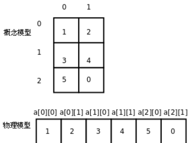
图 8.3. 多维数组
