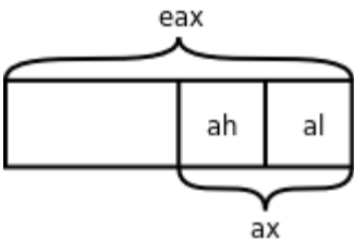
图 19.7. eax寄存器
