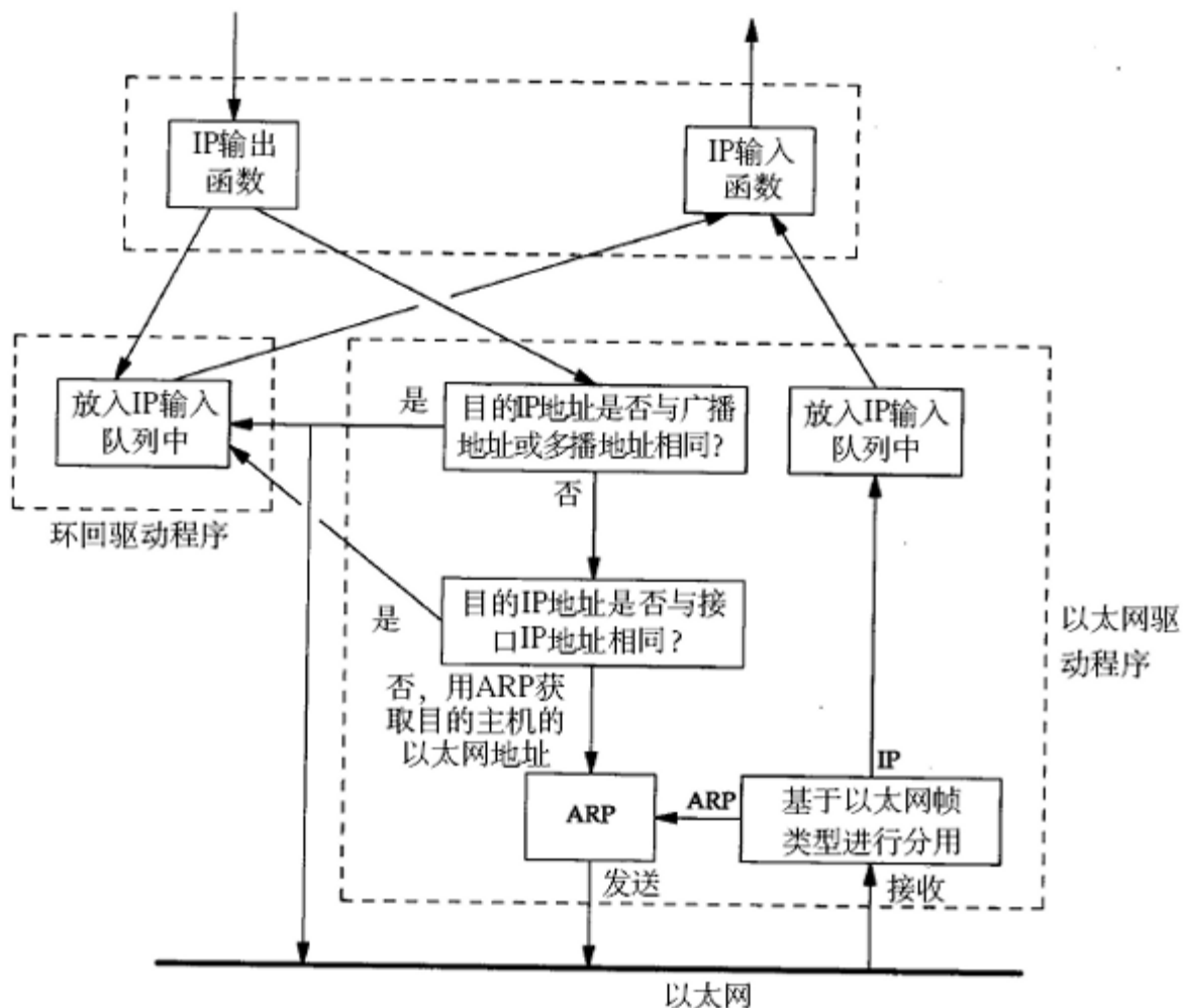
图 36.10. loopback设备
