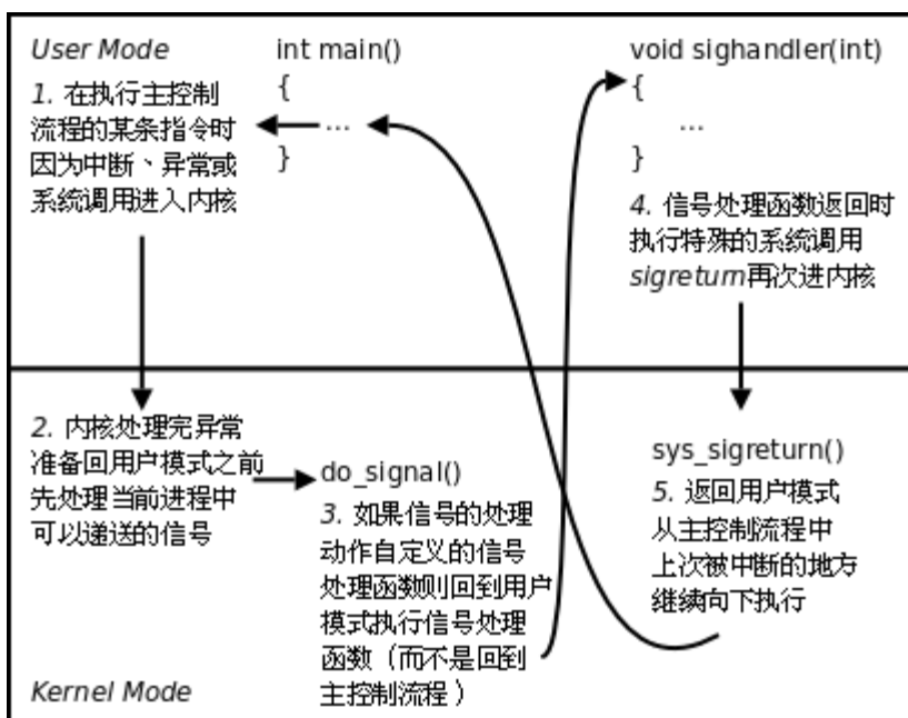
图 33.2. 信号的捕捉
