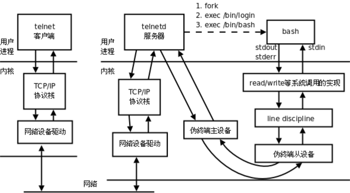
图 34.3. 伪终端
