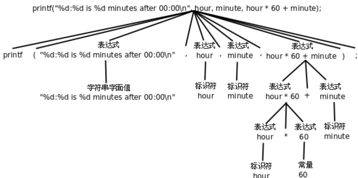
图 2.2. 语法树
