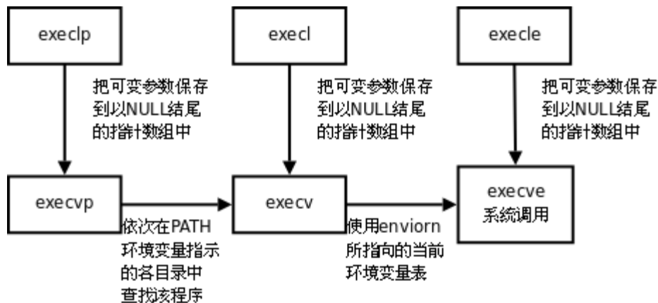
图 30.5. exec函数族
