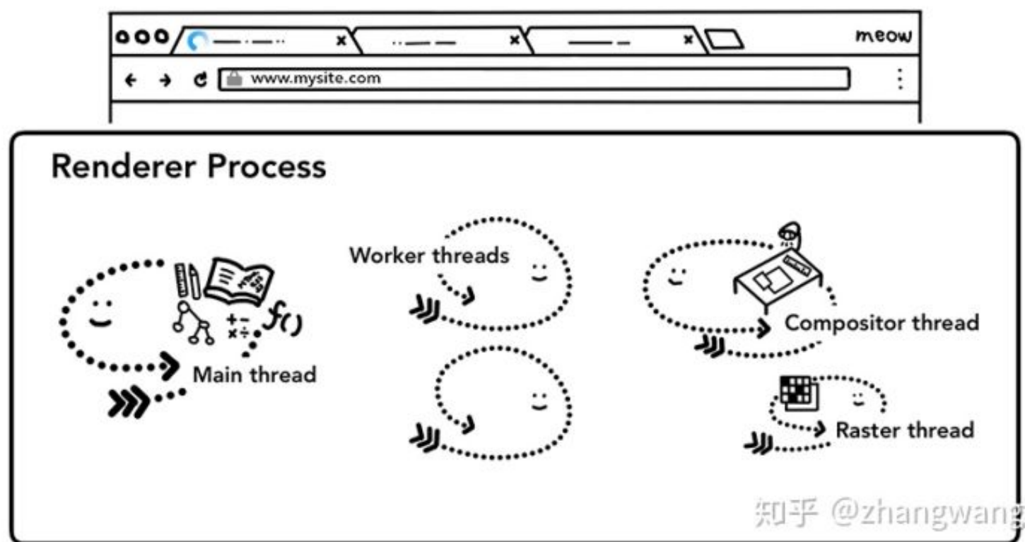
渲染进程包含的线程
