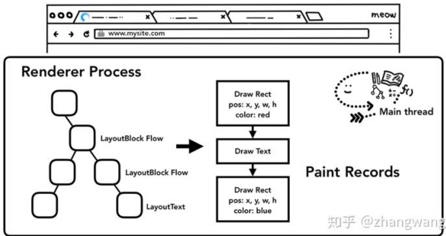
主线程依据布局树构建绘制记录
