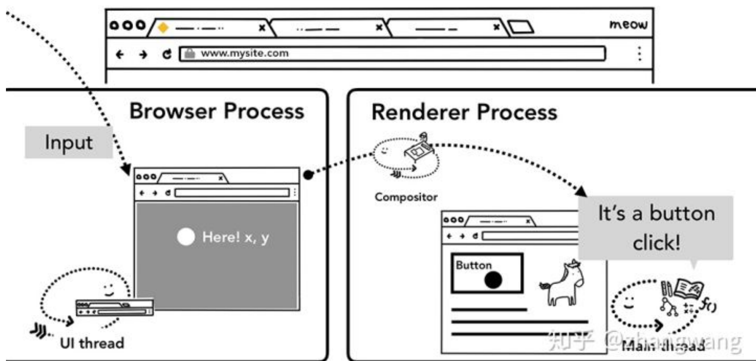
事件从浏览器进程传送给渲染进程
