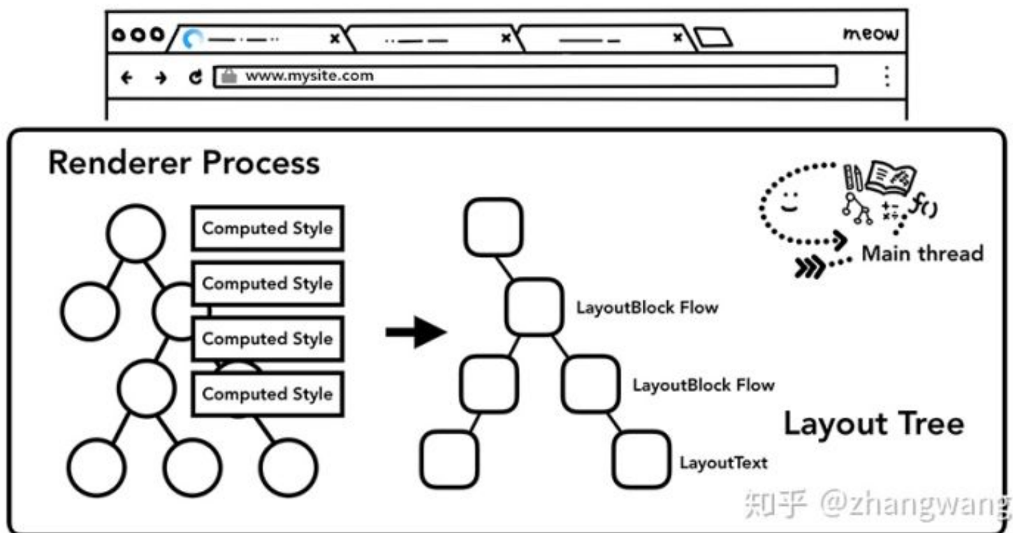
主线程遍历 DOM 及 对应元素的样式，构建出布局树
