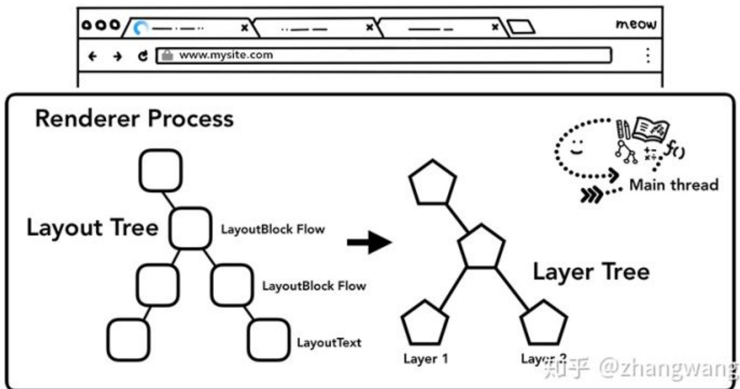
主线程遍历布局树生成层树
