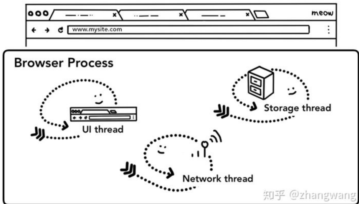
浏览器主进程中的不同线程
