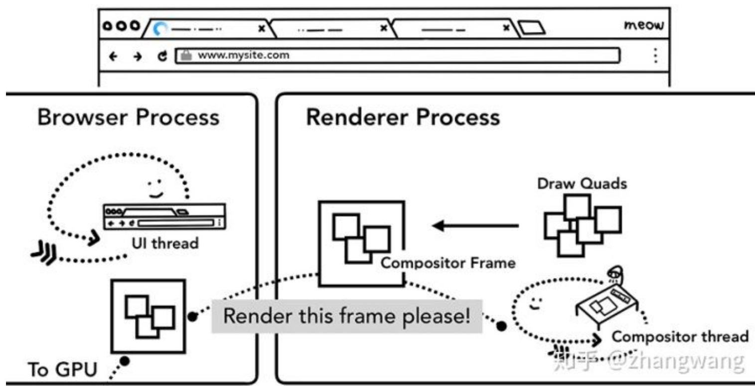
合成器线程会发送合成帧给 GPU 渲染
