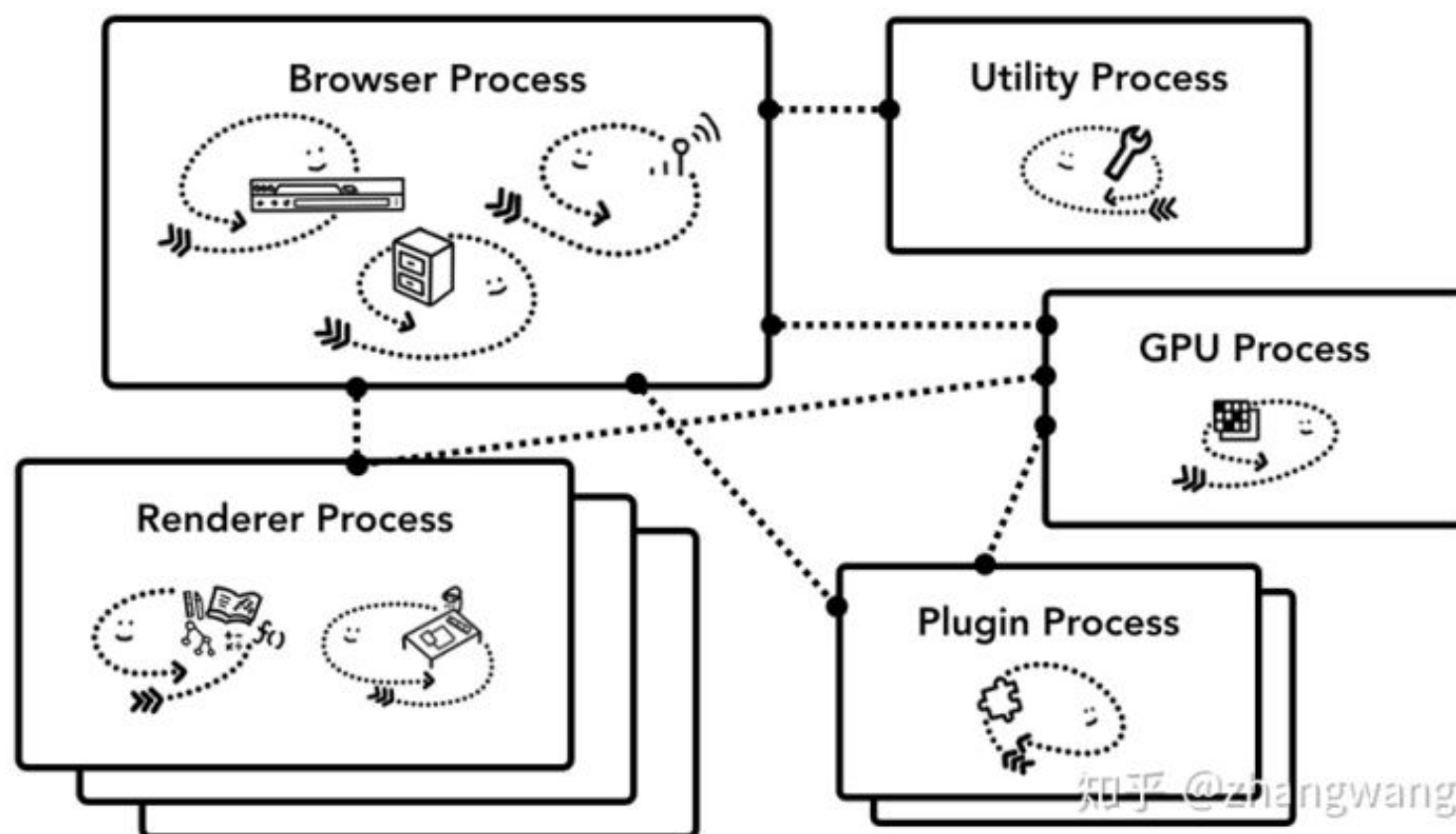
Chrome 的不同进程
