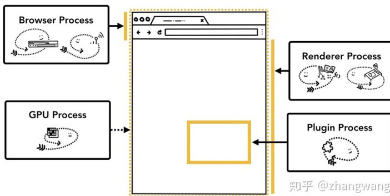
不同进程负责的浏览器区域示意图
