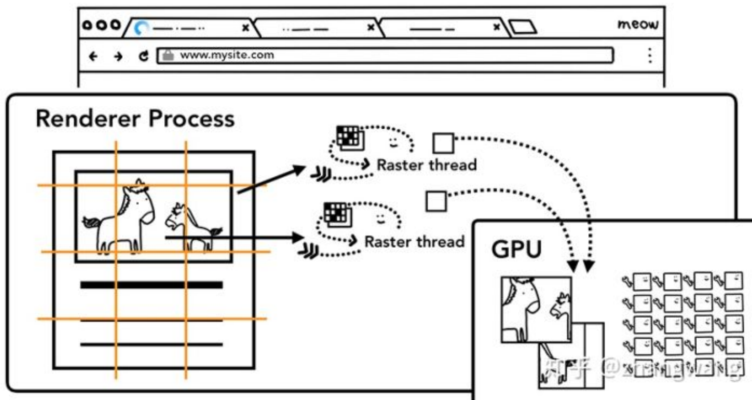
栅格线程会栅格化每一个磁贴并存储在 GPU 显存中
