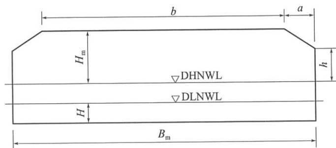
图 6-1 通航河流桥下通航净空示意图
