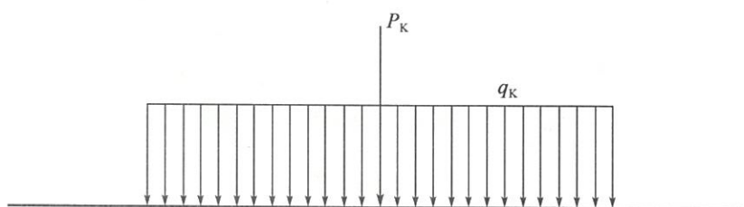
图 7.0.3 车道荷载
