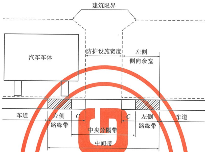
图 4-1 中间带示意图
